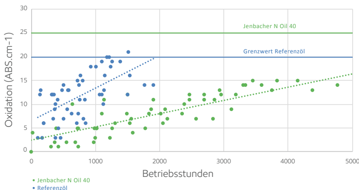
Oxidationsstabilität – Motor Baureihe 6F
